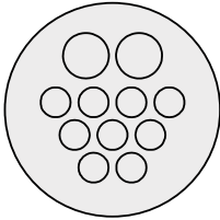
KEL-DP 32|11 A gy rund
