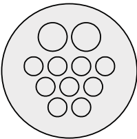
KEL-DP 32|11 B gy rund
